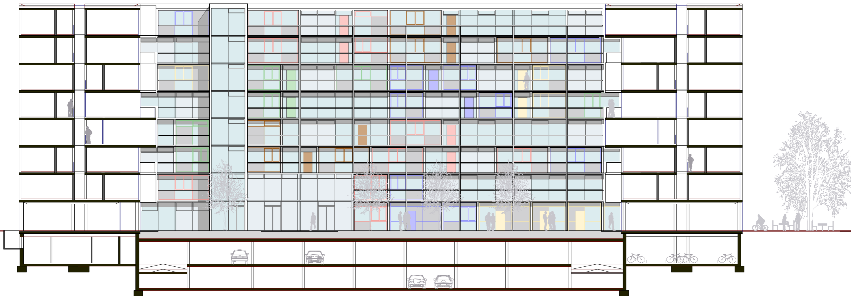
QUERSCHNITT/ANSICHT NORD - WESTEN m. 1 : 200
